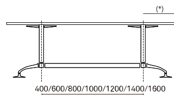
Larguero (medida entre ejes)
