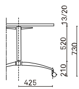
Pie largo con ruedas
