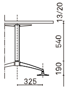
Pie corto con topes plástico
