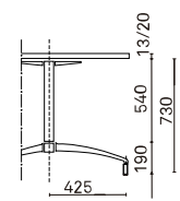
Pie largo con topes contract
