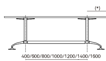
Larguero (medida entre ejes)
