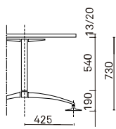
Pie largo con topes plástico
