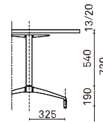
Pie corto con topes contract
