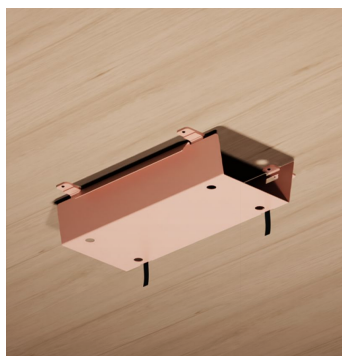
Goulotte Rabattable - AC099 / AC100 600x316xh126mm / 900x316xh126mm. Goulotte métallique rabattable pour logement d'électrification. Couleur personnalisable.
