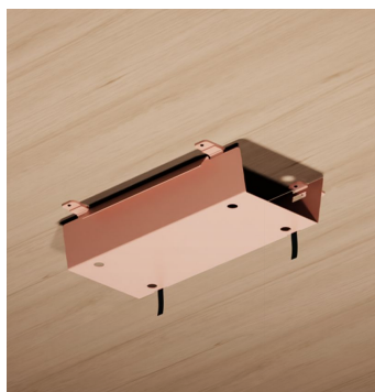
Bandeja Abatible - AC099 / AC100 600x316xh126mm / 900x316xh126mm. Bandeja metálica abatible para alojamiento de electrificación.
