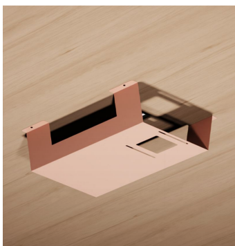
Bandeja Doble - AC078 600x460x154mm. Bandeja doble metálica para alojamiento de electrificación. Personalizable en color.
