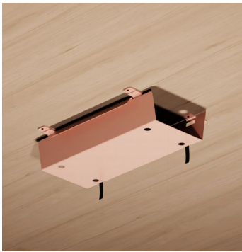
Bandeja Abatible - AC099 / AC100 600x316xh126mm / 900x316xh126mm. Bandeja metálica abatible para alojamiento de electrificación. Personalizable en color.
