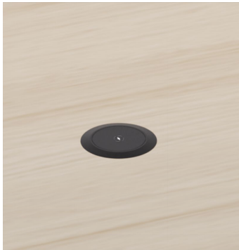
Multi chargeur Pro - AC085 Ø80mm en support / Ø71mm en découpe. Chargement sans fils + chargement USB A et C. Couleur noir.
